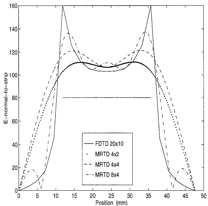
Figure 3: TEM E-pattern.
